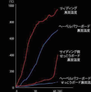
【外壁材裏面と内装せうこうボード裏面の温度変化】
