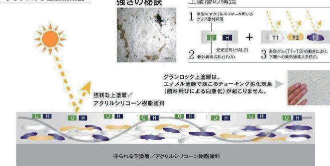
グランロック塗膜構成図
